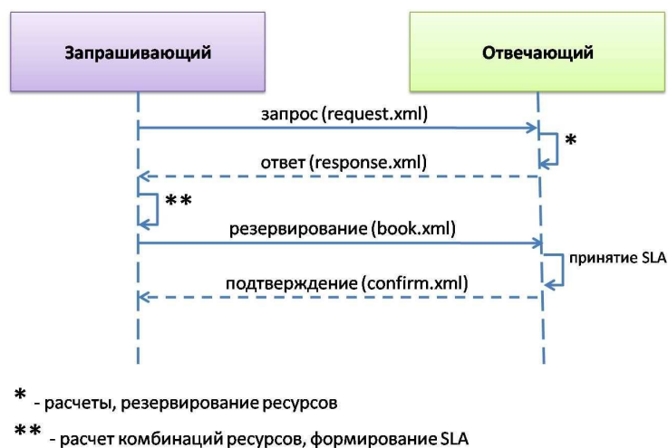
Рис. 3: Процесс подключения устройства к облачной инфраструктуре
