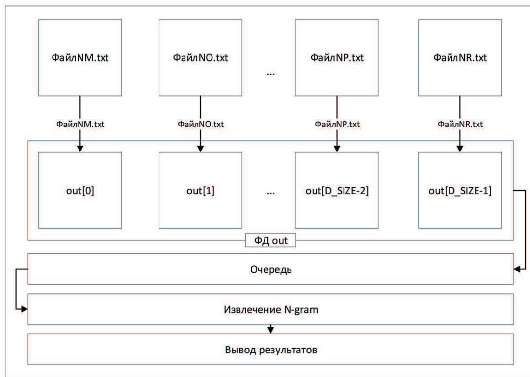
Рисунок 2 – Схема реализации алгоритма извлечение N-gram на ФВ
