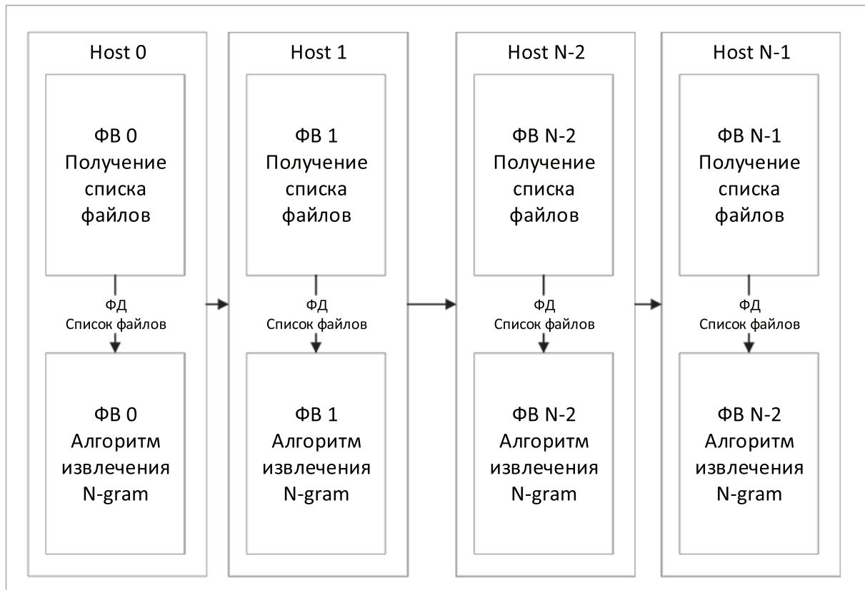
Рисунок 1 – Схема реализации алгоритма извлечения N-gram в системе LuNA
